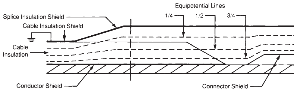
Fig. 8-4 Dielectric Field-Equipotential Lines-Tape Type Splice
