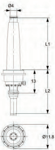
TEV 145/170 kV
