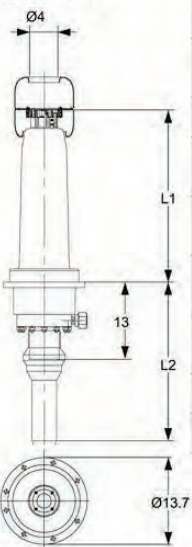
TEV 145/170 kV
